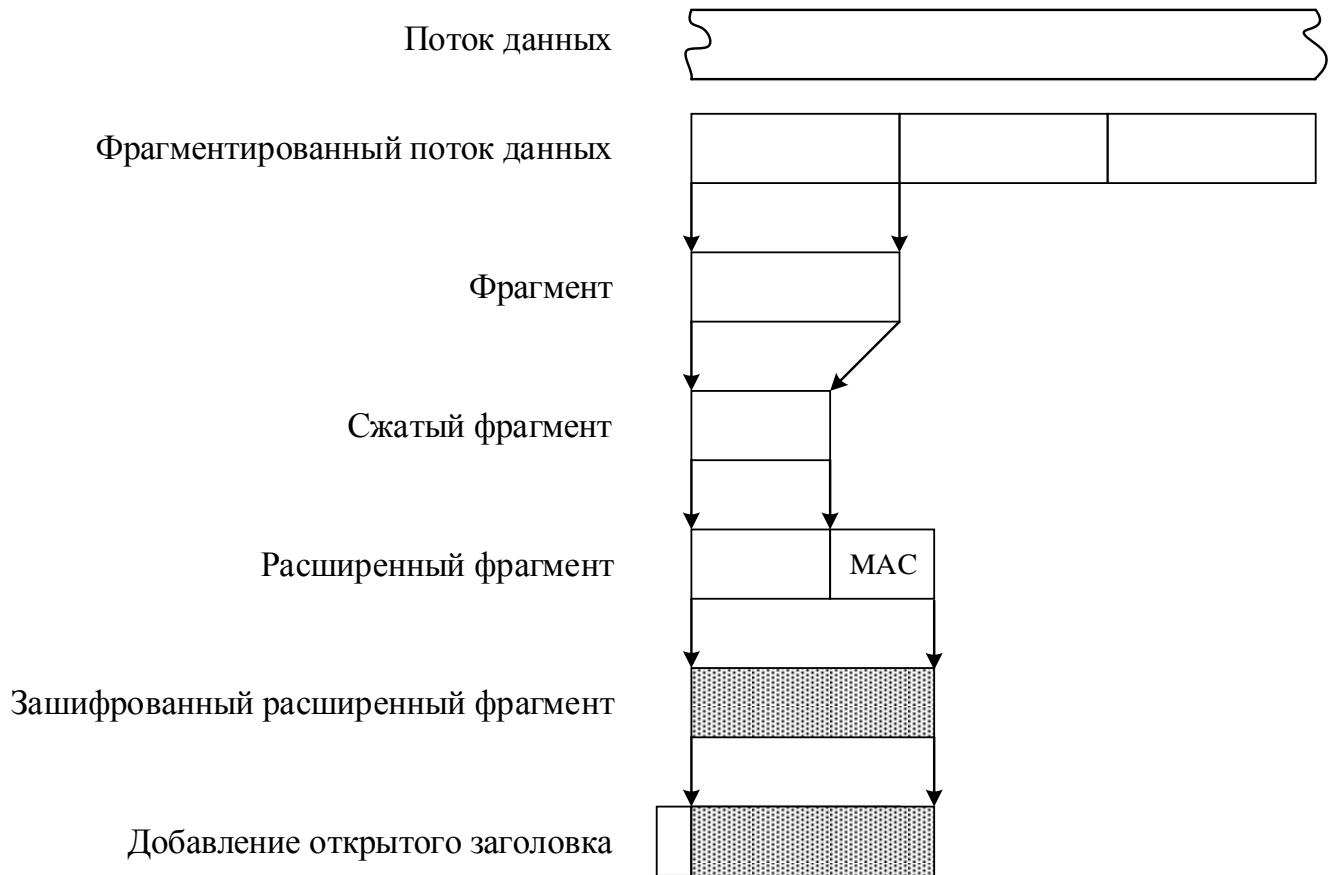
Рисунок 10.4.1 — Алгоритм преобразования информации при обмене с использованием протокола TLS
