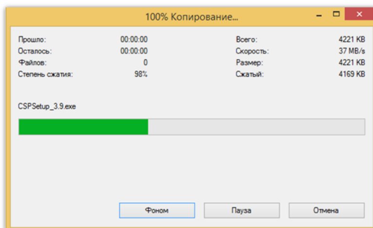
Рисунок 2. Процесс копирования
