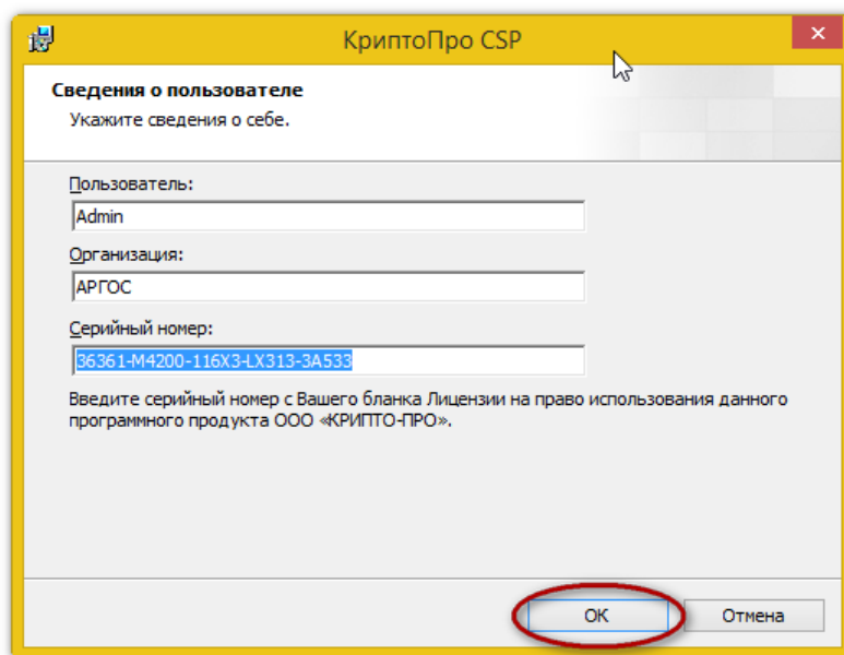
Рисунок 7. Ввод лицензии
