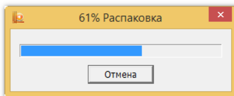
Рисунок 4. Распаковка
