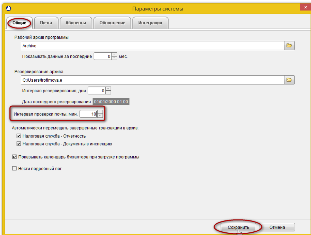
Рисунок 12. Настройка параметра автоматической проверки почты
