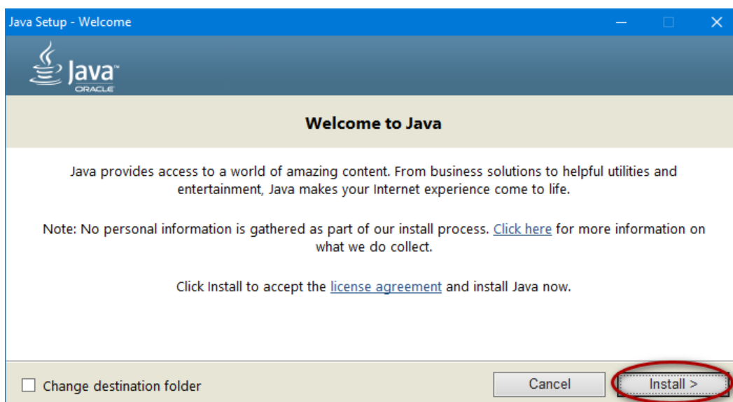
Рисунок 4. Установка Java
