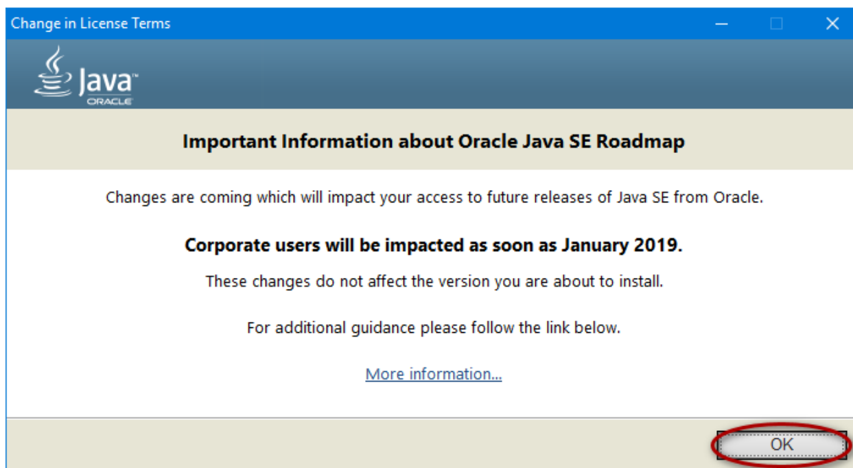
Рисунок 5. Установка Java
