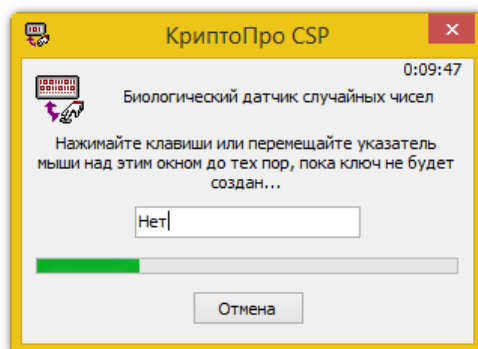
Рисунок 6. Генерация ключа
